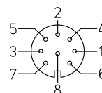
CONN-DIN-8F
