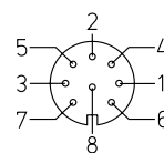
CONN-DIN-8F
