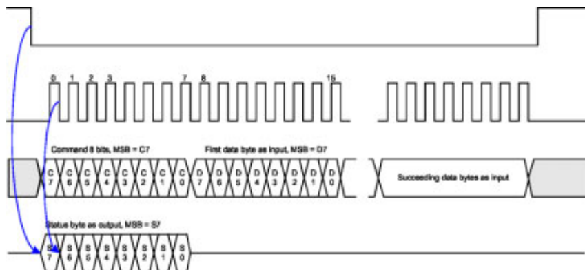
图 8 SPI 写操作
