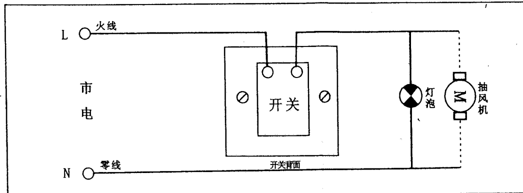
接线示意图
