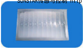
型号: 8719(幕帘式透镜) 焦距: 25 角度: 90° 距离: 10m 尺寸: 34 × 53.5
