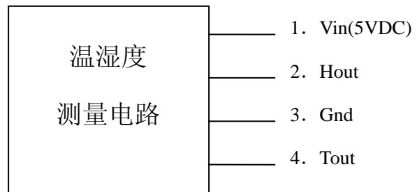
图 2. 接线实例.
