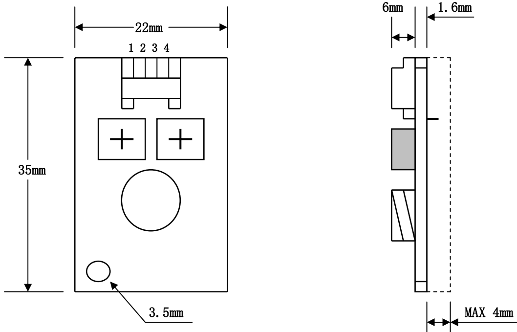
图 1. 外形图.
