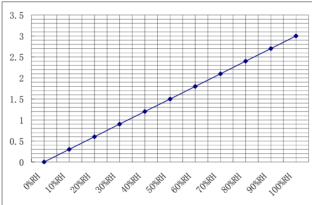
图 4. 标准特性图
