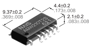
2 optocouplers type
