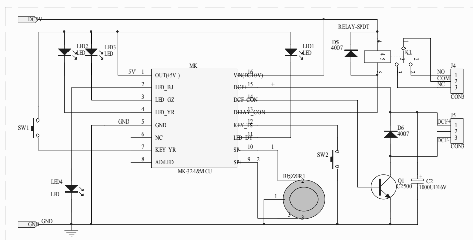
M402 推荐应用原理图
