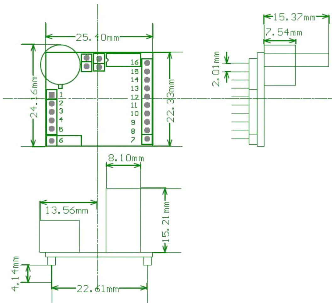
M402 引脚图
