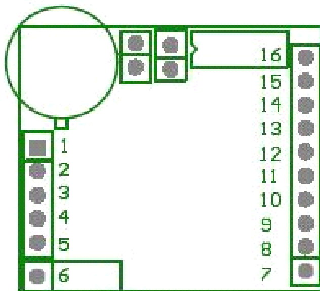
M402 引脚图
