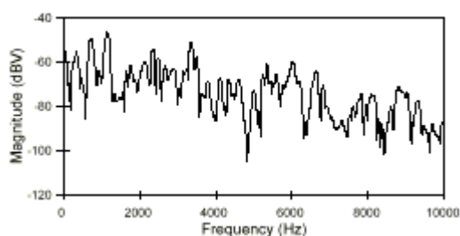
图 15:图 12 时间信号的 FFT 分析, 显示能量在宽频带上的分布
