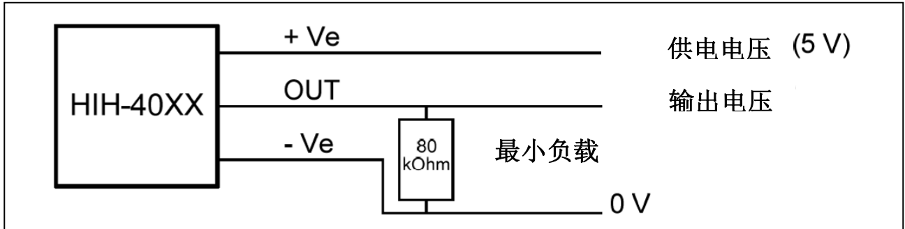
图 7. 典型应用电路
