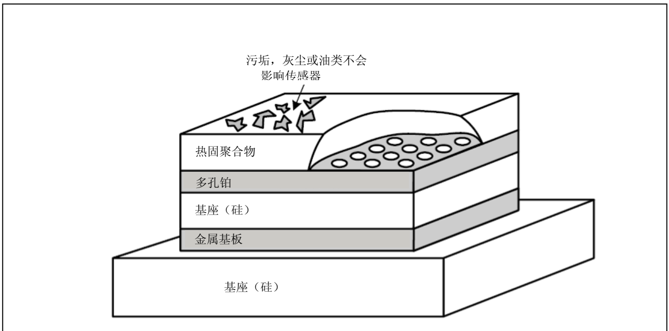
图 6. RH 传感器结构示意图
