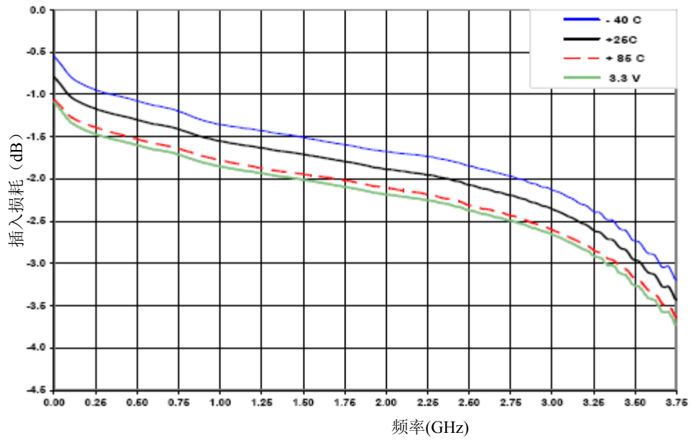
典型 AT4510 参考插入损耗
