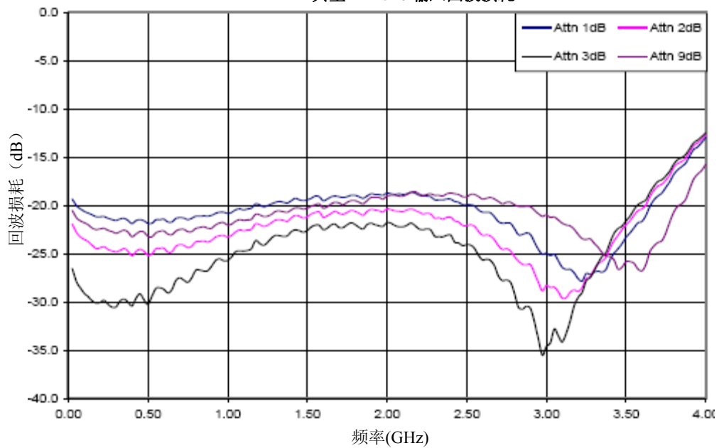
典型 AT4510 输入回波损耗
