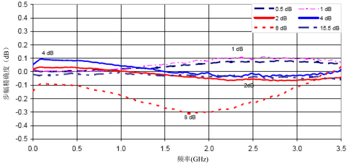
典型 AT4510 步幅精度
