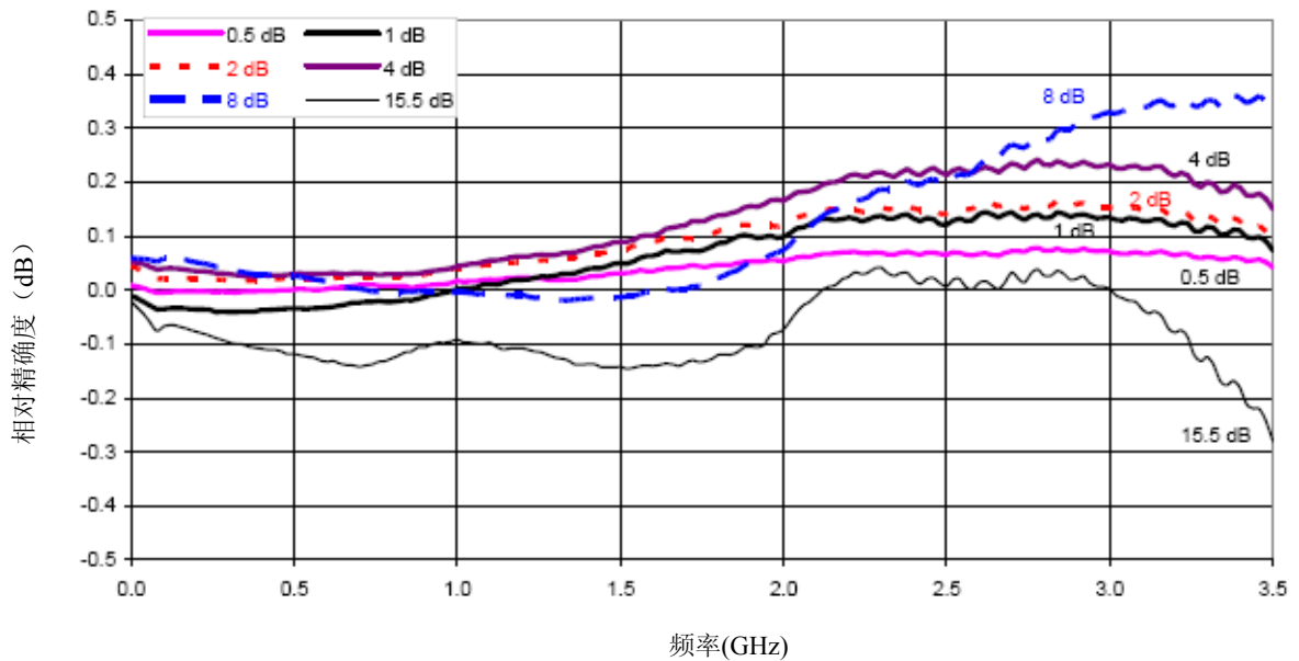
典型 AT4510 相对精度
